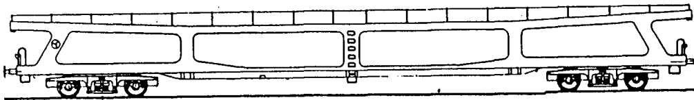
Typ DDM für Autoreisezüge, LÜP 22 cm
